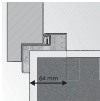
Ъглова каса МАЛА ПЛЮС
