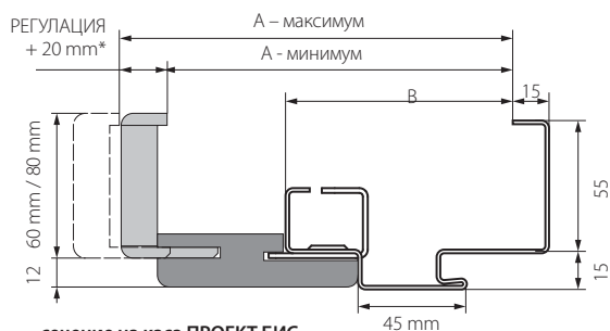
сечение на каса ПРОЕКТ БИС
