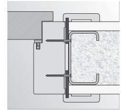
монтиране на винтове в стена от гипсокартон
