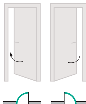
ВРАТИ С ОБРАТЕН ФАЛЦ ЛЯВО КРИЛО ДЯСНО КРИЛО
