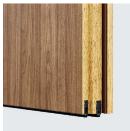
автоматични падащи прагове (вариант на касата на вратата ПОРТА СИСТЕМ)
