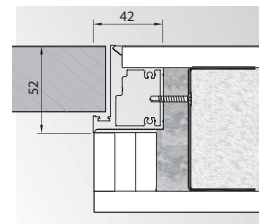
без фалц (отваряне навън)
