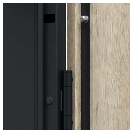
4 противовзломни болта
