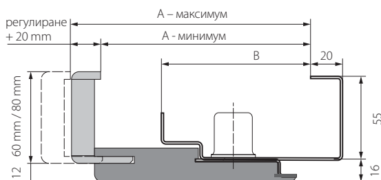
сечение на каса ПРОЕКТ Премиум
