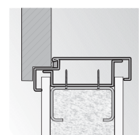
ГОЛЯМА ъглова каса монтаж на стена гипсокартон
