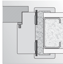
монтаж с пяна в стена от гипсокартон
